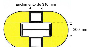
CP300 com enchimento de 310 mm
