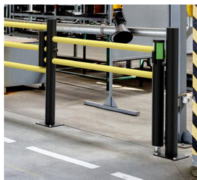
Porta “OSCAR” instalada em sistema “DELTA”
