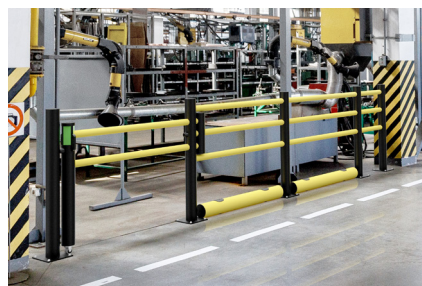
Porta “OSCAR” instalada em sistema “DELTA” + “MIKE”
