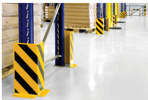
Protetores de Estantes com forma em L (Art. nº 6260)
